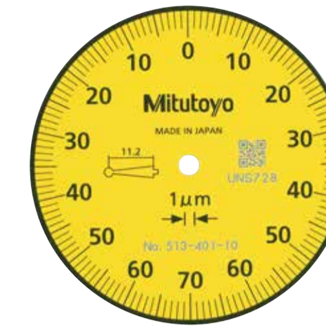
1 µm mittakaava-asteikko
