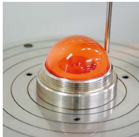
Exemple de vérification de la précision de rotation
