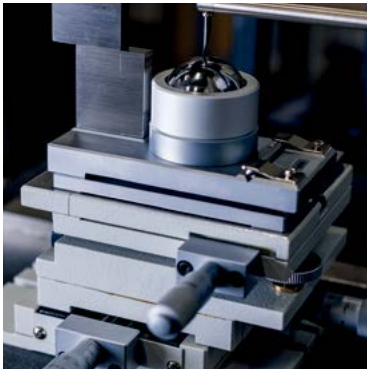
Exemple d'étalonnage du stylet
