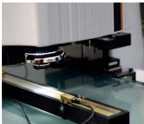
Exemples de mesure des axes X et Y
